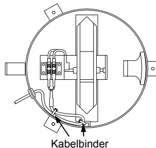
Abbildung 2: Aufgewickelte Kabel
