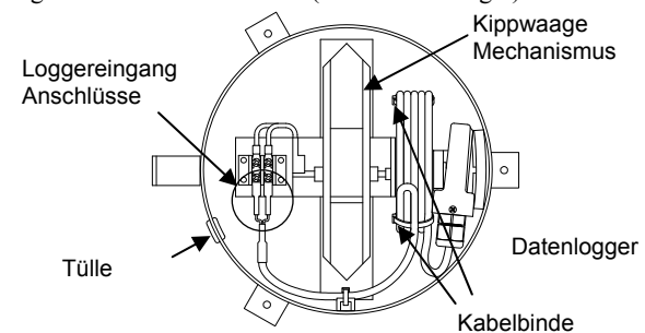
Abbildung 1: Regenmesser Innenansicht (Ring-, Sieb- und Trichteranordnung entfernt)
