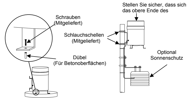
Abbildung 5: Oberflächenmontage
